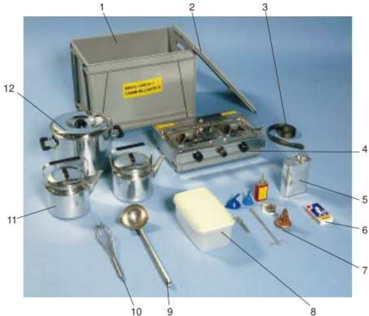
Bild 61. Varmhållningsutrustning /S
