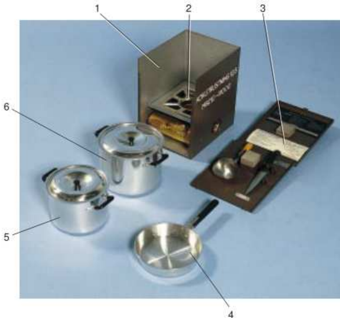
Bild 60. Kokustrustning 10 /S
