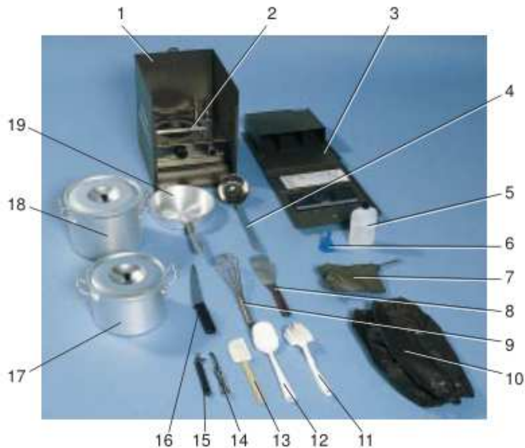
Bild 59. Kokutrustning 10 B /S
